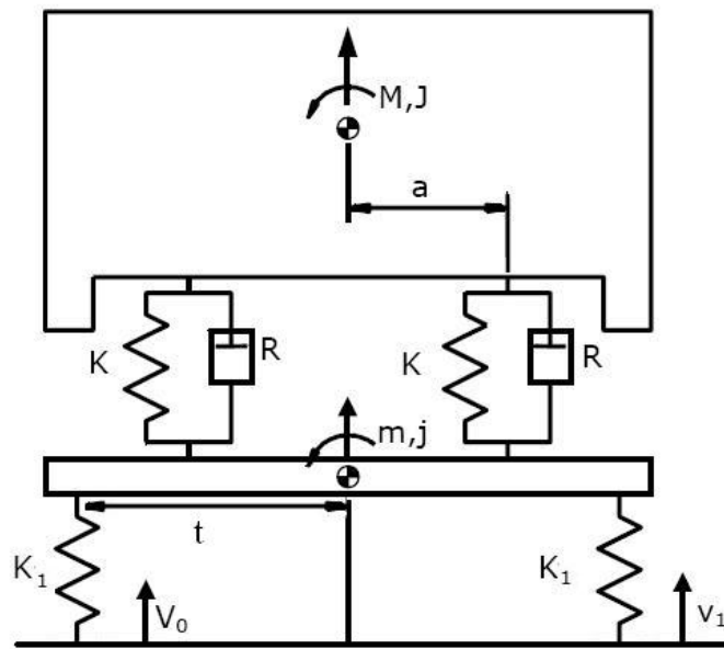
Figura 1. Modelo transversal del vehículo.
