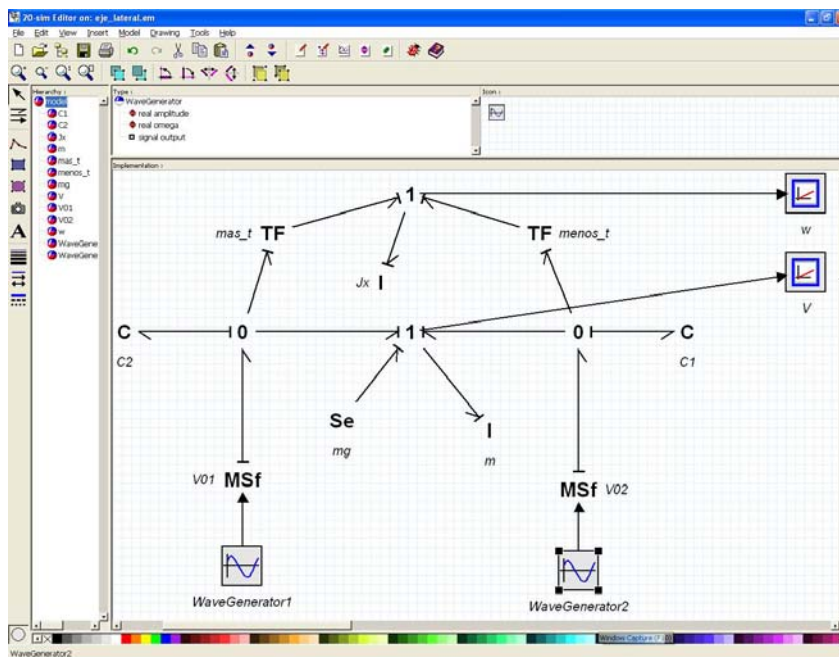
Figura 4. Implementación 20-Sim de eje del vehículo (vista transversal).
