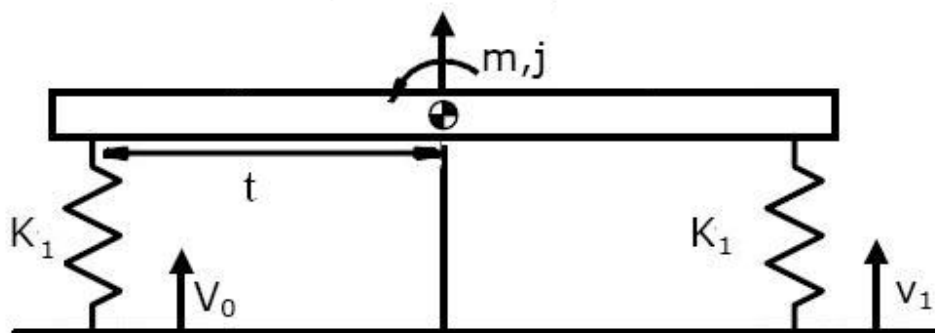
Figura 2. Eje del vehículo (vista transversal).
