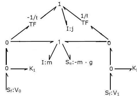
Figura 3. Diagrama Bond Graph del eje del vehículo.
