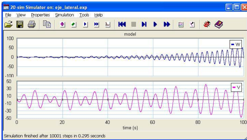
Figura 6. Comportamiento lateral si V_0 es distinta de cero.
